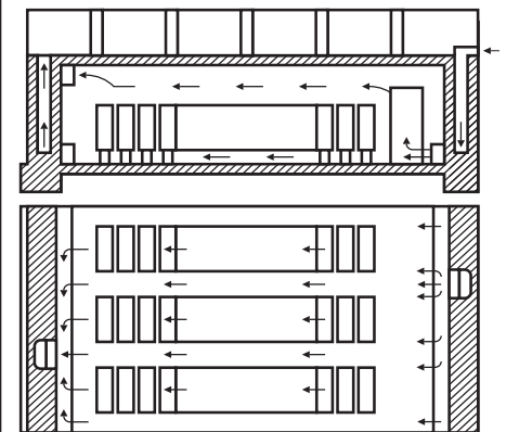
Рис. 4 Организация двусторонней естественной вентиляции.
