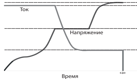
Рис. 3 Зависимость тока и напряжения заряда от времени в режиме IU, включая фазу заряда малым током и отключение батареи от зарядного устройства (IUa).
